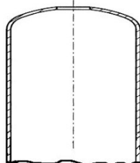
Чотири (4) витягування і одне пробивання
