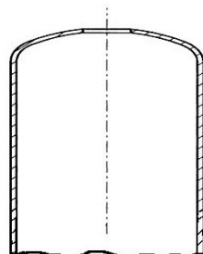
Два (2) витягування на одному обладнанні + пробивання
