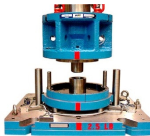
Два (2) витягування на одному обладнанні + пробивання
